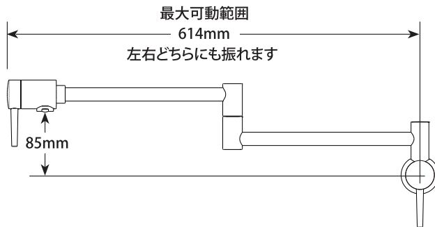
正面最大
