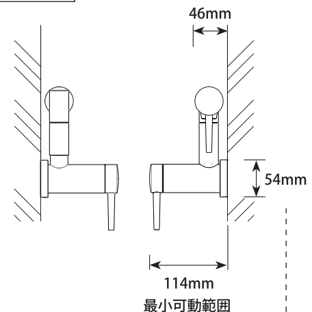
断面最小
